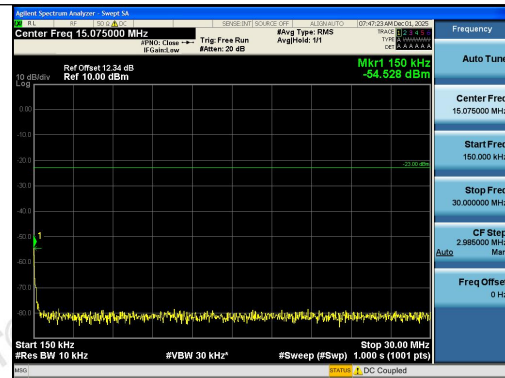
Band26(824-849)-10MHz-QPSK-26840-1RB#0-0. 15~30-PASS
