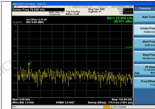
Band26(824-849)-10MHz-QPSK-26840-1RB#0-0. 009~0.15-PASS
