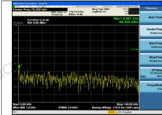
Band26(824-849)-10MHz-QPSK-26990-1RB#0-0. 009~0.15-PASS
