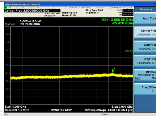
Band26(824-849)-10MHz-QPSK-26990-1RB#49-1 000~3000-PASS
