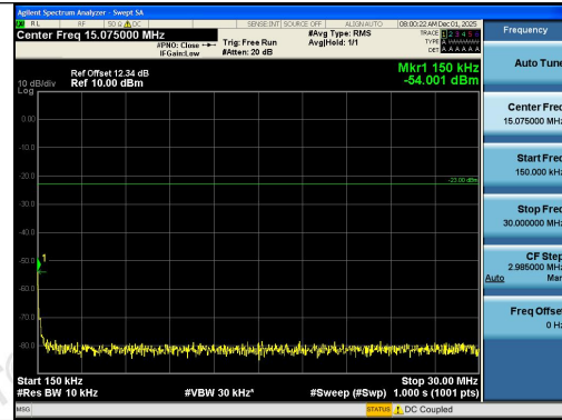
Band26(824-849)-10MHz-QPSK-26990-1RB#0-0. 15~30-PASS
