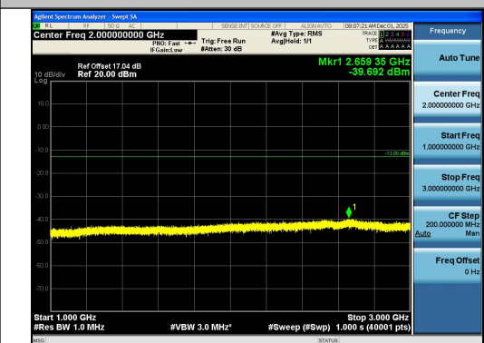
Band26(824-849)-10MHz-QPSK-26840-50RB#0-1 000~3000-PASS
