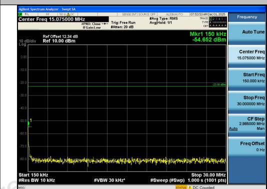
Band26(824-849)-10MHz-QPSK-26915-1RB#0-0. 15~30-PASS
