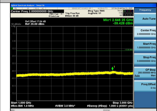
Band26(824-849)-10MHz-QPSK-26915-1RB#0-10 00~3000-PASS
