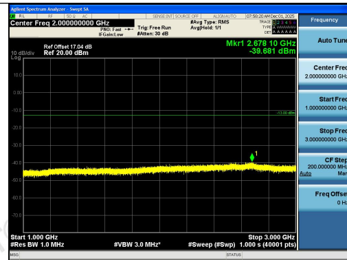
Band26(824-849)-10MHz-QPSK-26915-1RB#49-1 000~3000-PASS
