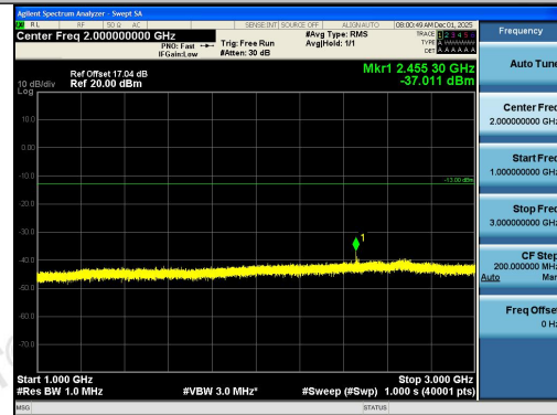
Band26(824-849)-10MHz-QPSK-26990-1RB#0-10 00~3000-PASS
