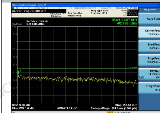
Band41-5MHz-QPSK-40620-25RB#0-0.009~0.15 -PASS
