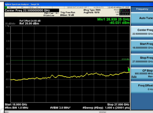
Band41-15MHz-QPSK-39725-1RB#0-18000~2700 0-PASS
