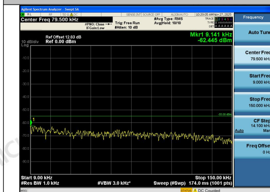
Band41-10MHz-QPSK-39700-50RB#0-0.009~0.15-PASS
