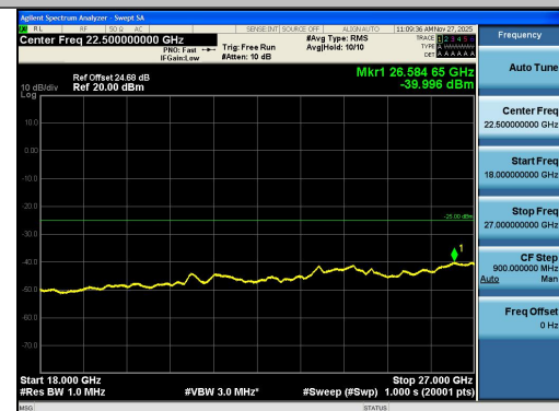
Band41-15MHz-16QAM-41515-1RB#74-18000~27 000-PASS
