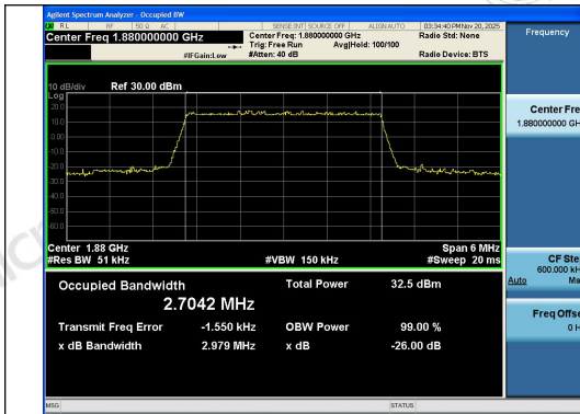
Band2-3MHz-QPSK-18900-15RB#0-PASS
