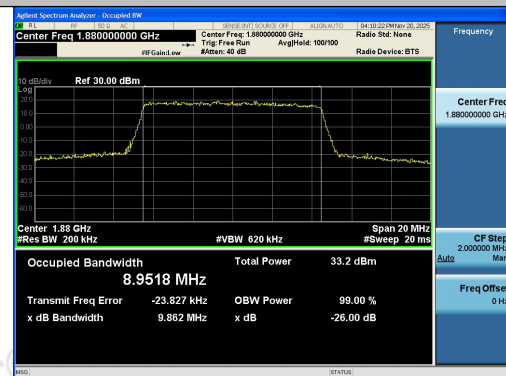
Band2-10MHz-QPSK-18900-50RB#0-PASS
