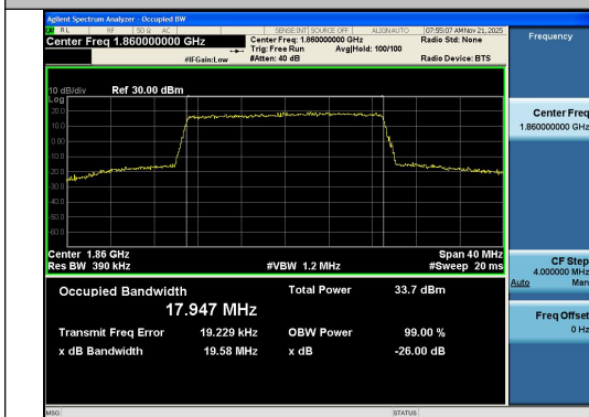
Band2-20MHz-QPSK-18700-100RB#0-PASS
