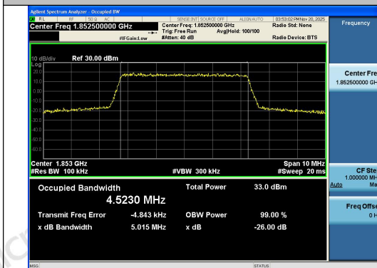
Band2-5MHz-QPSK-18625-25RB#0-PASS
