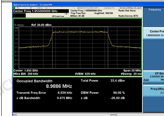
Band2-10MHz-QPSK-18650-50RB#0-PASS
