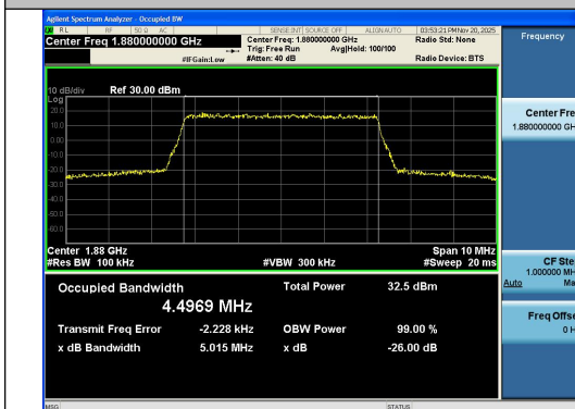
Band2-5MHz-QPSK-18900-25RB#0-PASS
