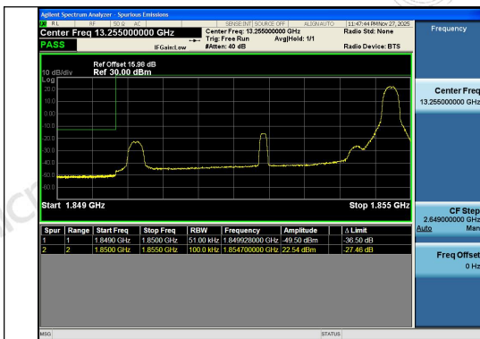
Band2-5MHz-QPSK-18625-1RB#24-PASS
