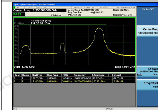
Band2-3MHz-QPSK-19185-1RB#14-PASS
