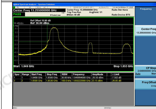
Band2-3MHz-QPSK-18615-1RB#0-PASS
