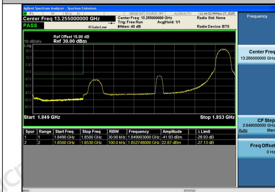
Band2-3MHz-QPSK-18615-1RB#14-PASS
