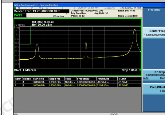
Band2-10MHz-QPSK-18650-1RB#49-PASS
