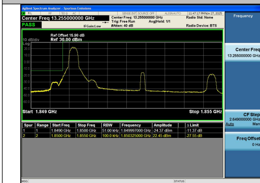
Band2-5MHz-QPSK-18625-1RB#0-PASS
