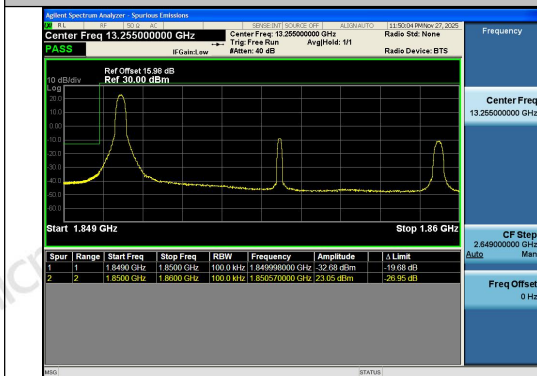
Band2-10MHz-QPSK-18650-1RB#0-PASS
