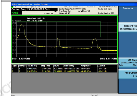
Band2-5MHz-QPSK-19175-1RB#0-PASS
