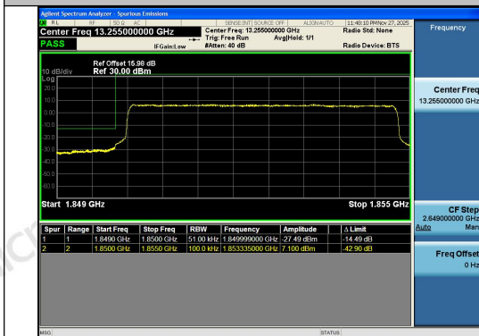
Band2-5MHz-QPSK-18625-25RB#0-PASS
