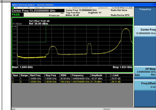
Band2-3MHz-16QAM-18615-1RB#14-PASS
