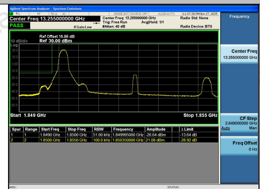
Band2-5MHz-16QAM-18625-1RB#0-PASS
