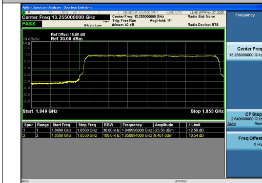
Band2-3MHz-QPSK-18615-15RB#0-PASS
