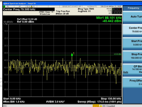
Band4-1.4MHz-QPSK-19957-1RB#0-0.009~0.15-
