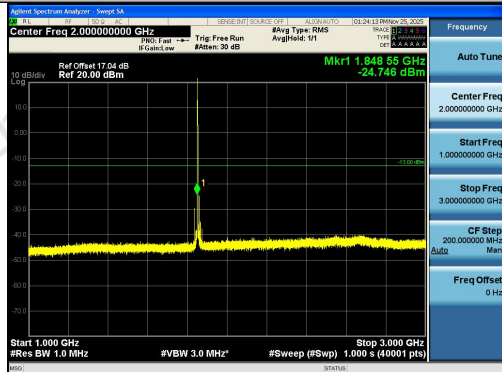
Band2-20MHz-16QAM-18700-1RB#0-1000~3000-
