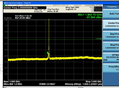
Band2-20MHz-QPSK-18700-1RB#99-1000~3000-
