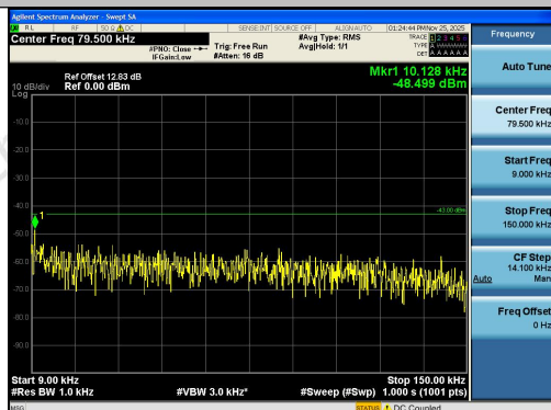
Band2-20MHz-QPSK-18700-1RB#99-0.009~0.15-
