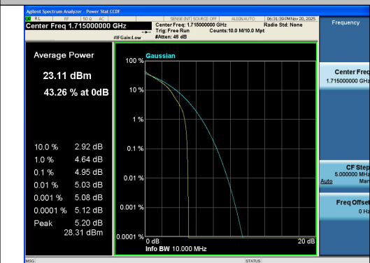
Band4-10MHz-QPSK-20000-1RB#0-PASS
