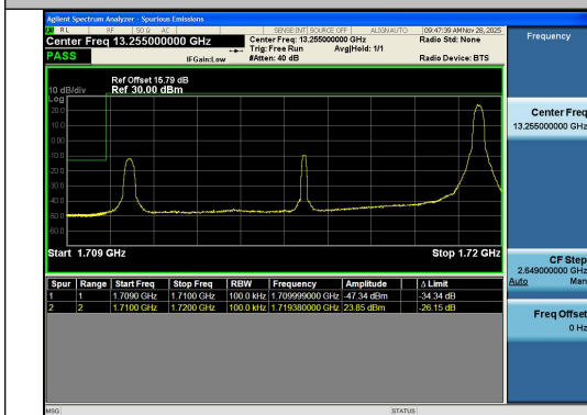
Band4-10MHz-QPSK-20000-1RB#49-PASS
