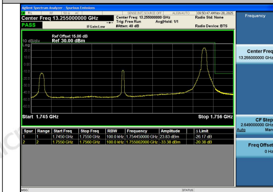
Band4-10MHz-QPSK-20350-1RB#49-PASS
