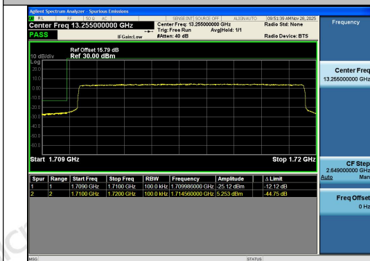
Band4-10MHz-QPSK-20000-50RB#0-PASS
