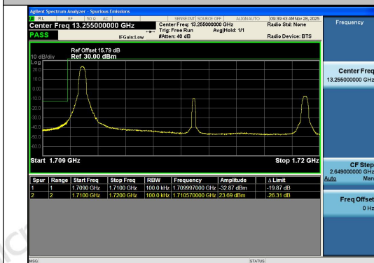
Band4-10MHz-QPSK-20000-1RB#0-PASS
