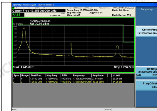
Band4-10MHz-QPSK-20350-1RB#0-PASS
