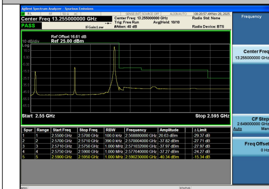
Band7-20MHz-QPSK-21350-1RB#99-PASS
