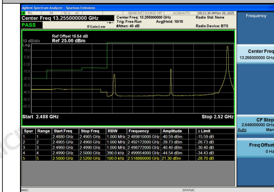
Band7-20MHz-QPSK-20850-1RB#99-PASS
