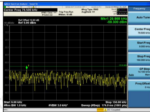
Band7-20MHz-QPSK-21350-100RB#0-0.009~0.15 -PASS
