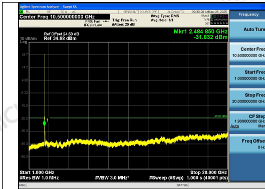
Band7-10MHz-QPSK-20800-50RB#0-1000~2000 0-PASS
