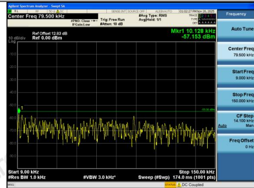
Band7-20MHz-QPSK-20850-100RB#0-0.009~0.15 -PASS
