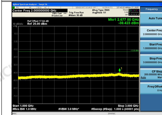
Band12-1.4MHz-QPSK-23173-6RB#0-1000~3000 -PASS
