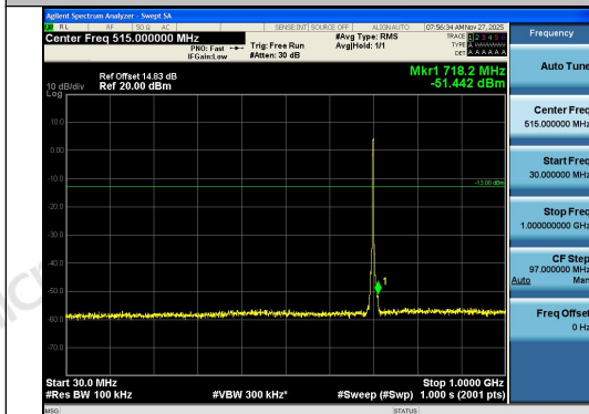
Band12-3MHz-QPSK-23095-15RB#0-30~1000-P ASS
