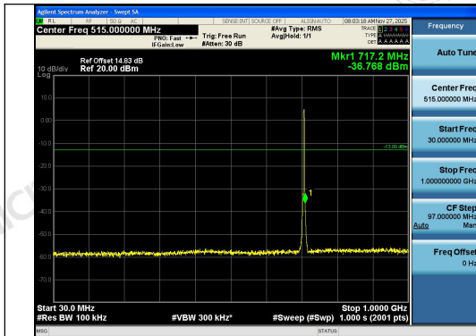
Band12-3MHz-QPSK-23165-15RB#0-30~1000-P ASS
