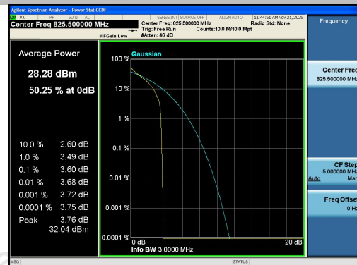
Band26(824-849)-3MHz-QPSK-26805-1RB#0-PA SS
