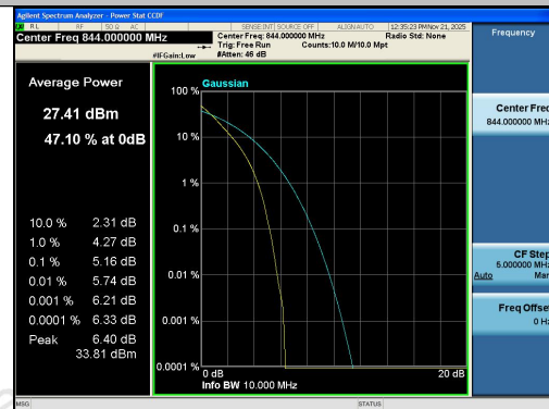
Band26(824-849)-10MHz-QPSK-26990-50RB#0-P
