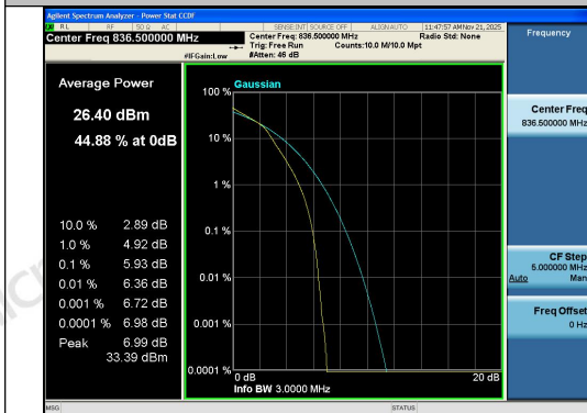
Band26(824-849)-3MHz-16QAM-26915-15RB#0-P ASS
