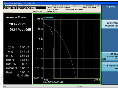
Band26(824-849)-3MHz-QPSK-26915-1RB#0-PA SS
