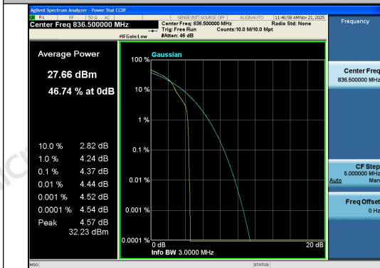
Band26(824-849)-3MHz-16QAM-26915-1RB#0-P ASS
