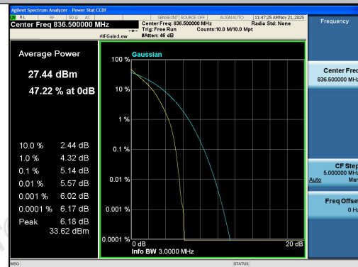
Band26(824-849)-3MHz-QPSK-26915-15RB#0-P ASS
