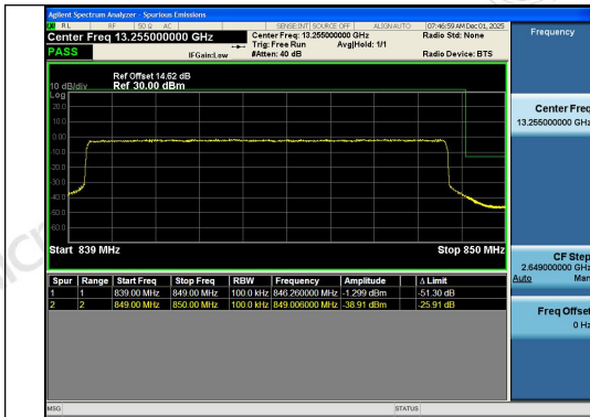
Band26(824-849)-10MHz-QPSK-26990-50RB#0-P
