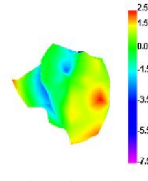
2500.000MHz E1
