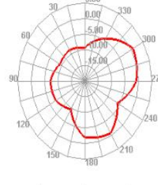
2500.000MHz E2
