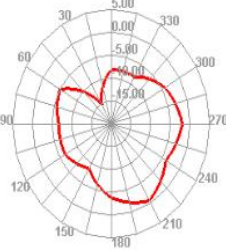
2400.000MHz E2
