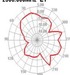
2500.000MHz E1
