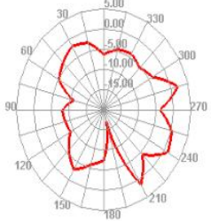
2400.000MHz E1
