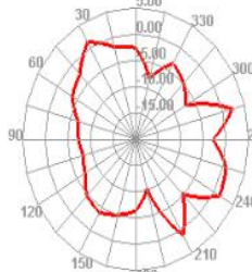
2450.000MHz E1
