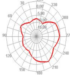
2450.000MHz E2
