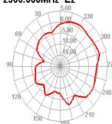
2500.000MHz E2
