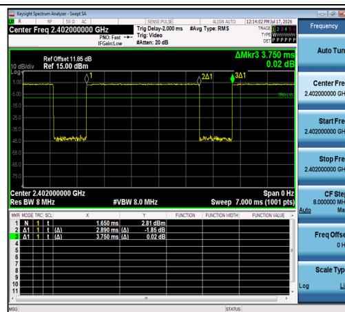
NTNV-2DH5-Ant1-2402
