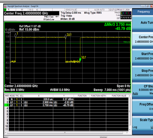
NTNV-2DH5-Ant1-2480
