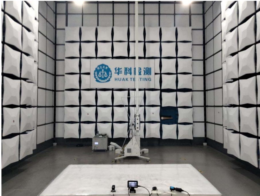
Model: F1 Radiated Emissions
