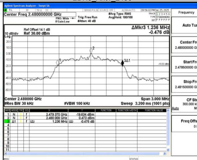
2DH5_Ant1_2480
