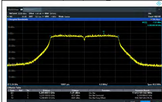
11ac (HT20) CH48_99%
