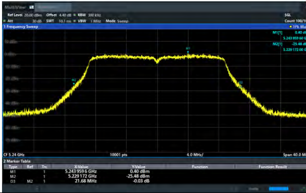
11n (HT20) CH48_26dB
