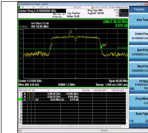
11n40ISO-Ant1-5510
