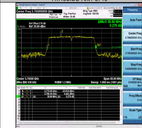
11n40ISO-Ant1-5795
