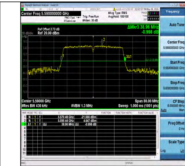
11n40ISO-Ant1-5590
