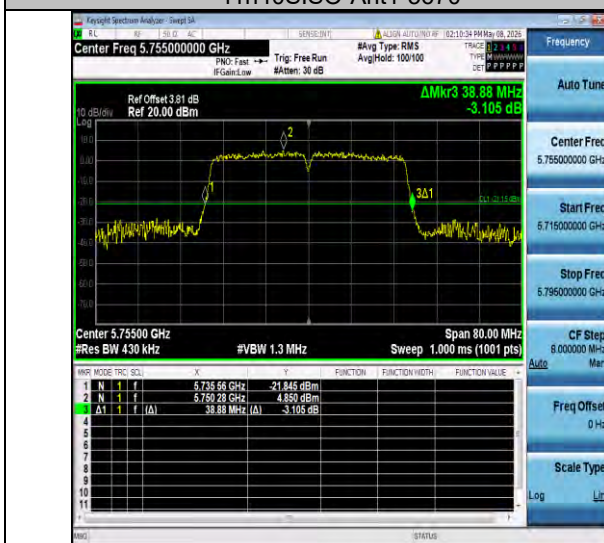
11n40ISO-Ant1-5755
