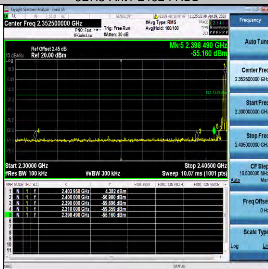
3D5-Ant1-Hop 2402-PASS
