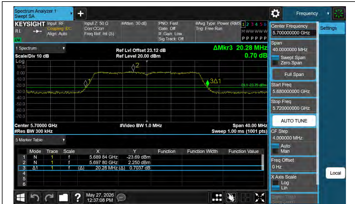
11N20MIMO-Ant2-5700
