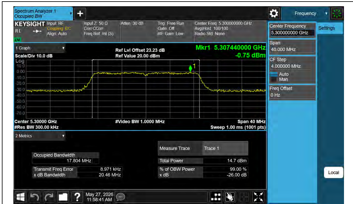
11N20MIMO-Ant2-5300
