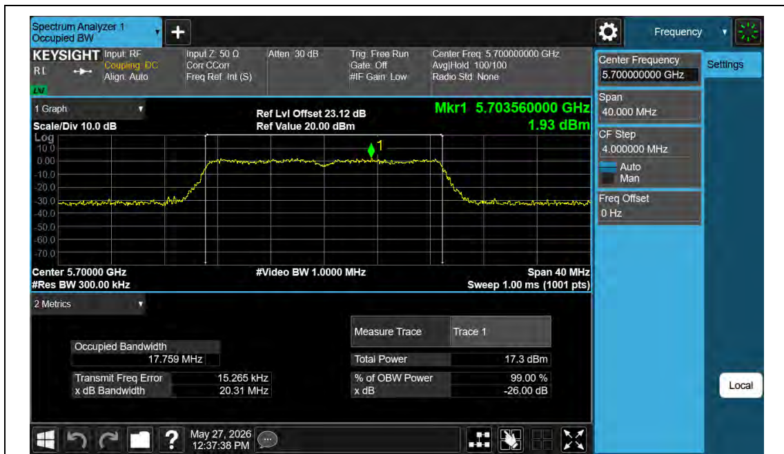
11N20MIMO-Ant2-5700
