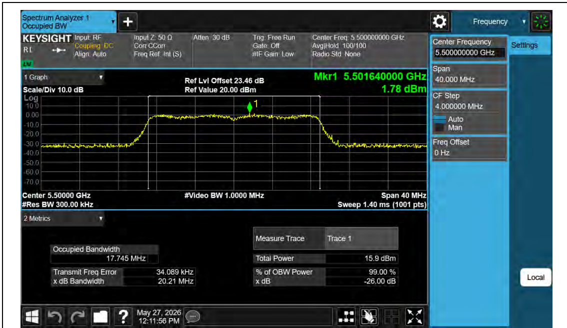
11N20MIMO-Ant2-5500
