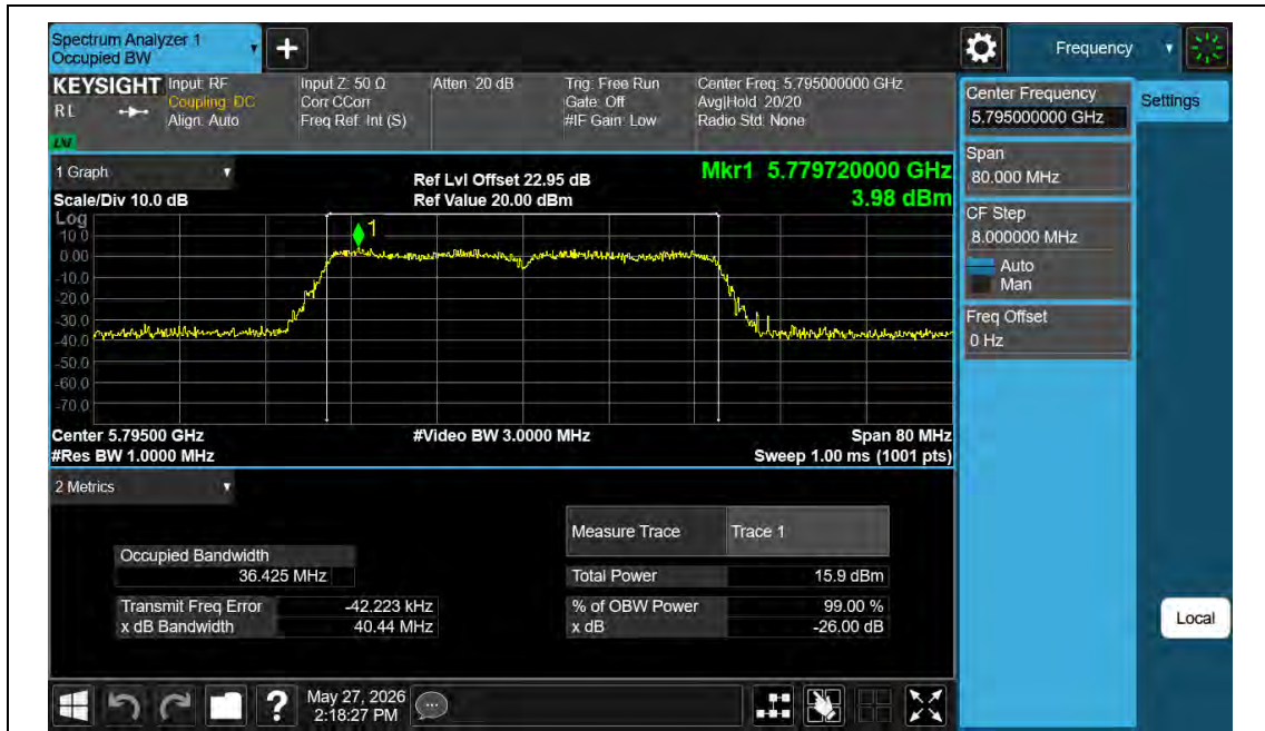
11N40MIMO-Ant2-5795
