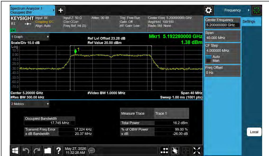
11N20MIMO-Ant2-5200
