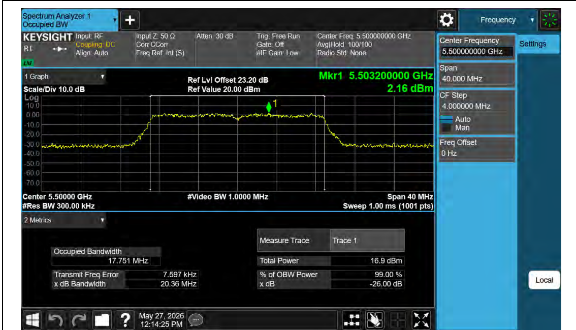
11N20MIMO-Ant1-5580
