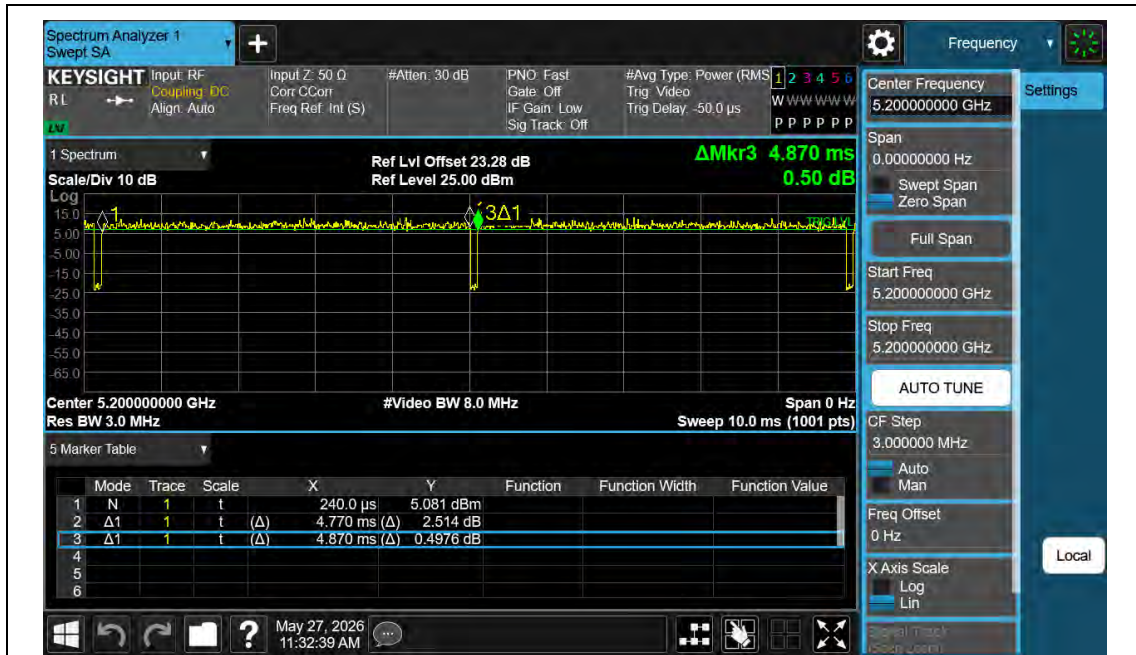
NTNV-11N20MIMO-Ant2-5200
