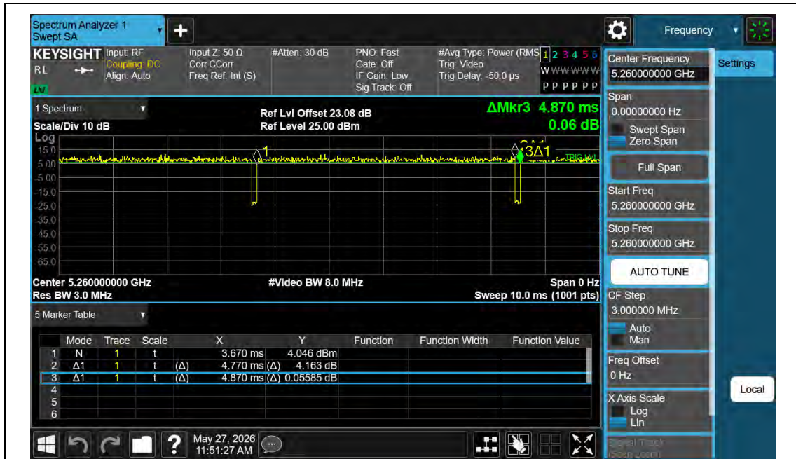
NTNV-11N20MIMO-Ant2-5260
