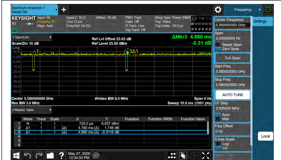
NTNV-11N20MIMO-Ant1-5700
