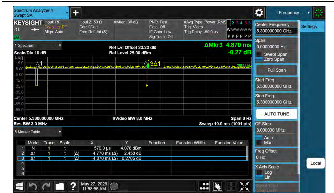
NTNV-11N20MIMO-Ant2-5300
