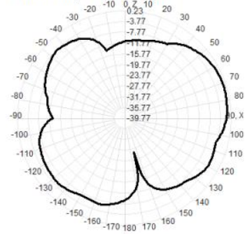
2400.0MHz Total(E1-XZ), Max=-0.99dBi
