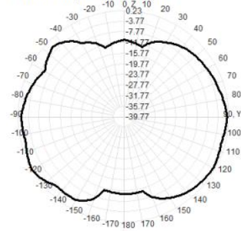
2400.0MHz Total(E2-YZ), Max=0.23dBi
