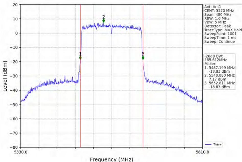
802.11ax(HEW160)_MCH_5570MHz_2xRU996_Left_Ant1_NTNV
