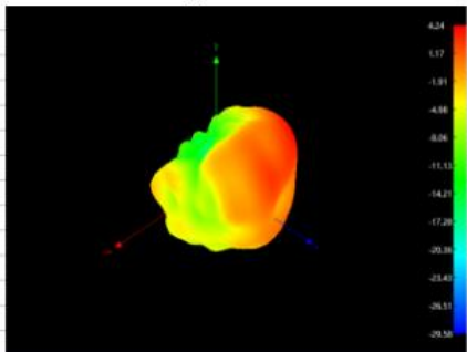
5000MHz
