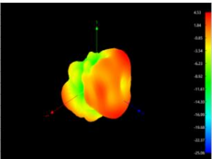
5500MHz
