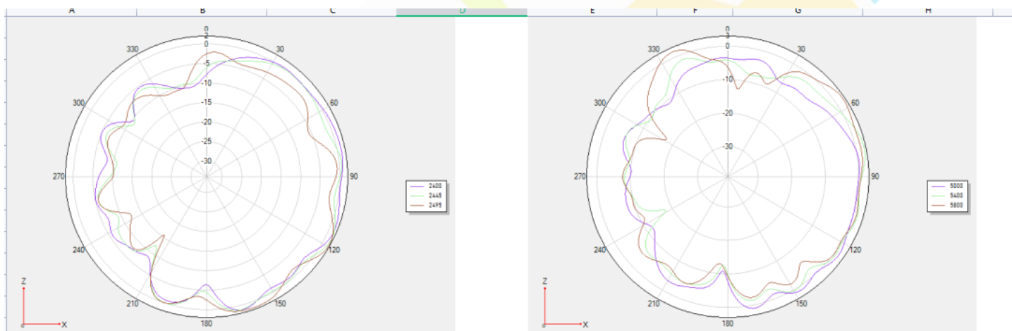
Phi 0 2D图
