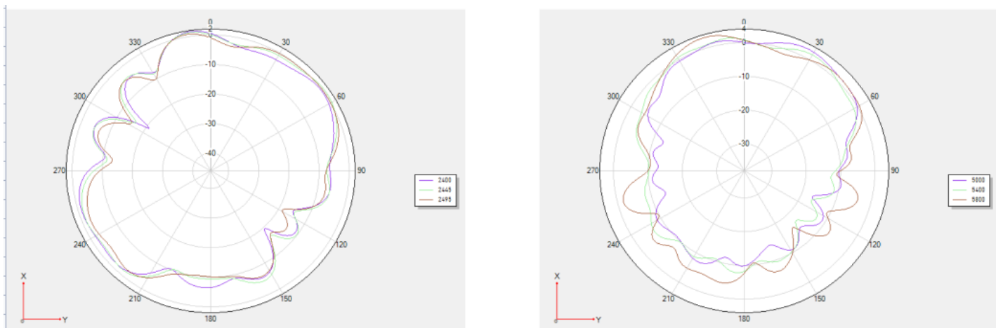
Theta 90 2D图
