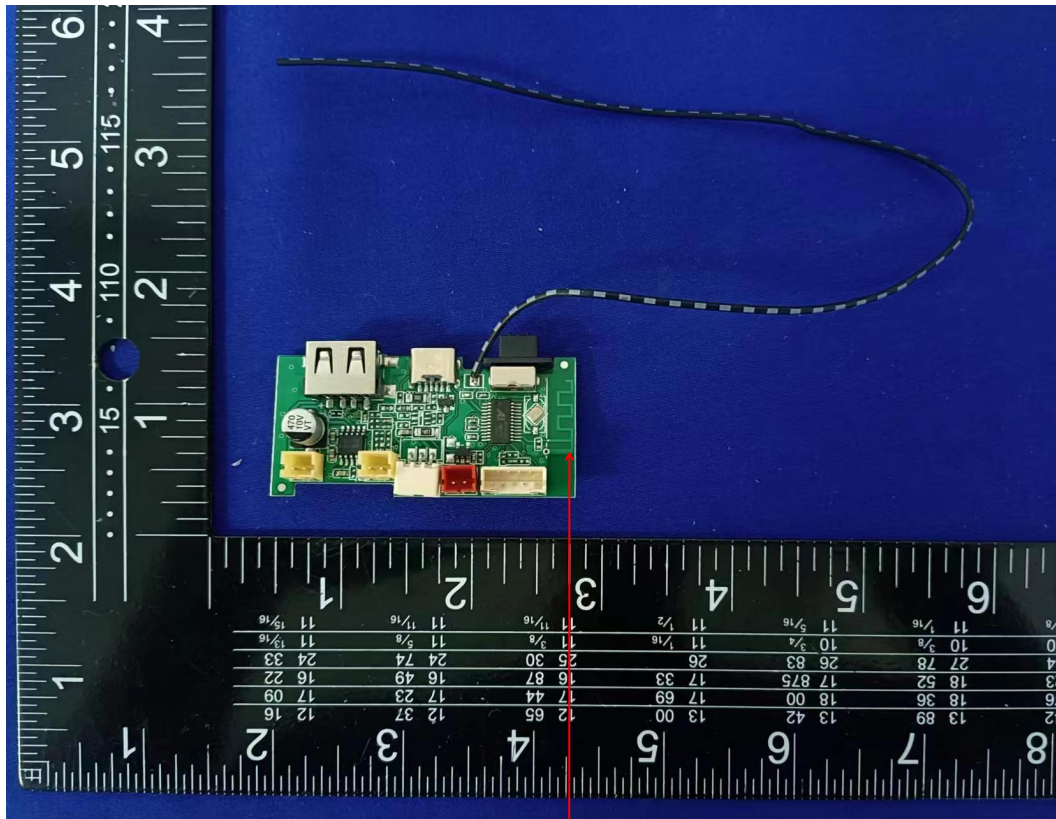
PCB ANT
