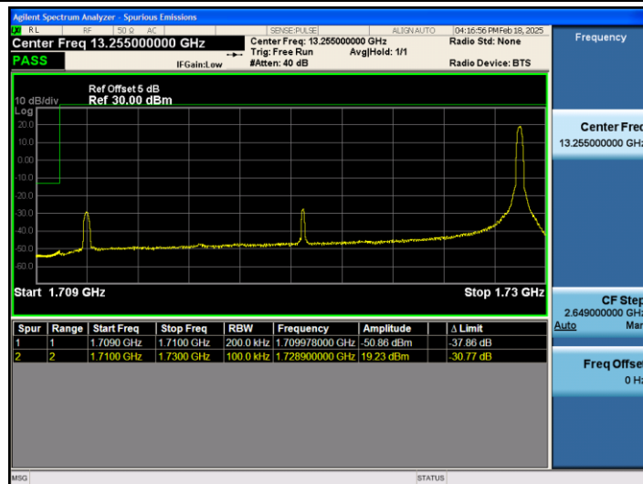
Band66_20MHz_QPSK_132072_1RB#99
