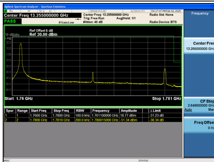
Band66_20MHz_QPSK_132572_1RB#0
