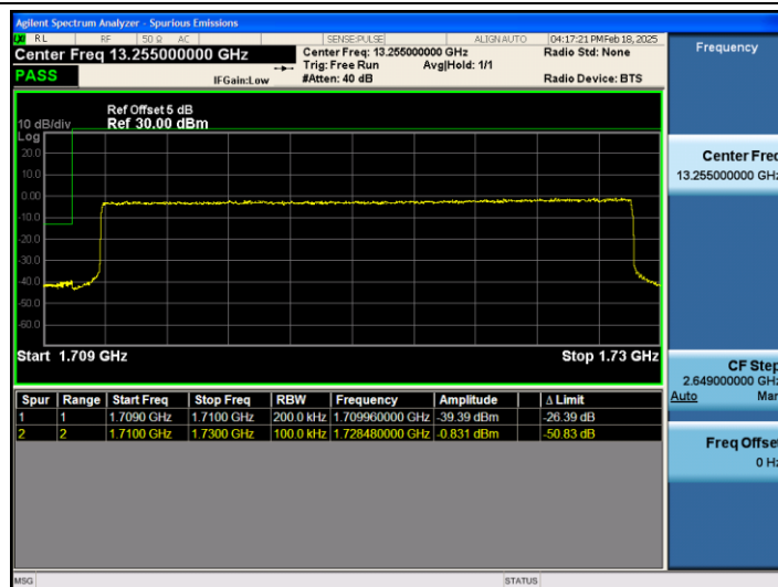
Band66_20MHz_QPSK_132072_100RB#0
