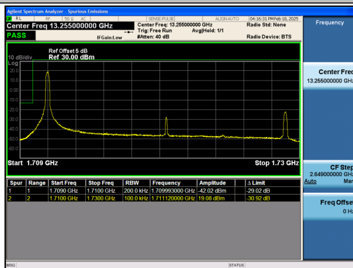
Band66_20MHz_QPSK_132072_1RB#0
