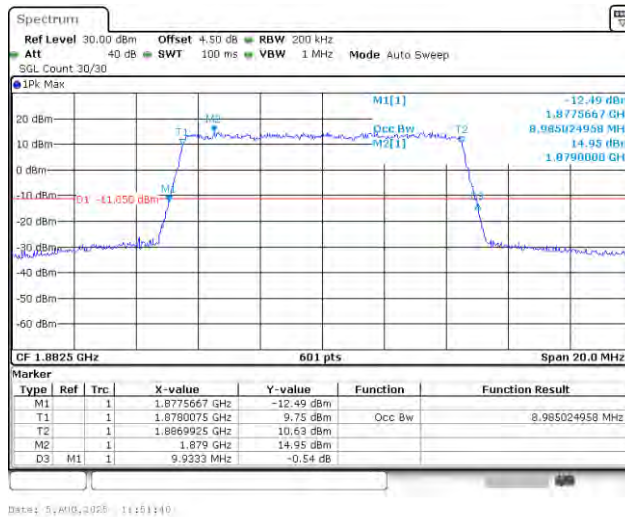
Band25-10MHz-QPSK-26365-50RB#0-PASS
