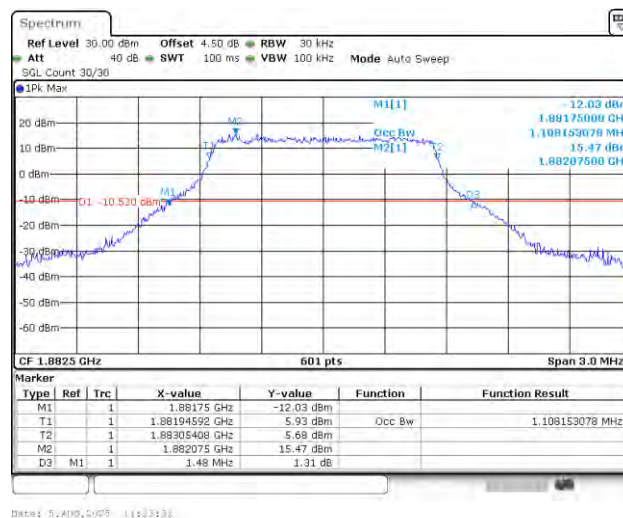
Band25-1.4MHz-QPSK-26365-6RB#0-PASS
