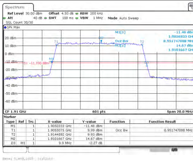
Band25-10MHz-QPSK-26640-50RB#0-PASS
