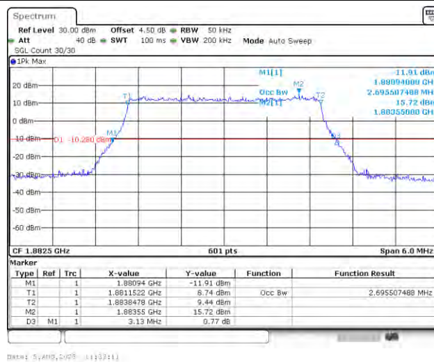
Band25-3MHz-QPSK-26365-15RB#0-PASS
