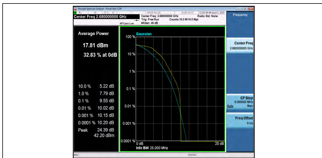
Band41-20MHz-QPSK-41490-1RB#0-PASS
