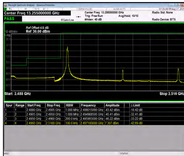
Band41_20MHz_QPSK_39750_1RB#0
