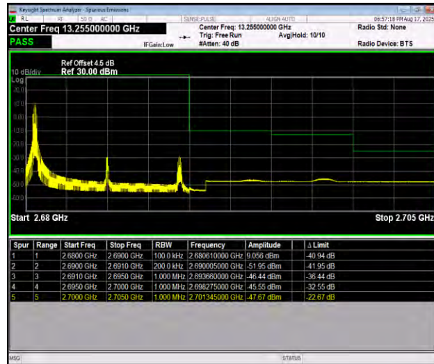
Band41_10MHz_QPSK_41540_1RB#0
