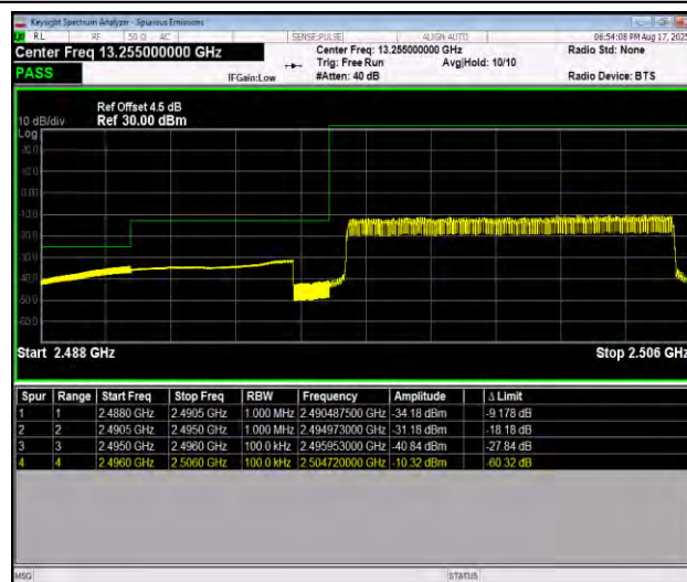
Band41_10MHz_QPSK_39700_50RB#0
