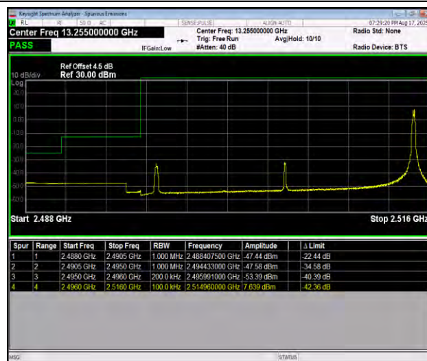
Band41_20MHz_QPSK_39750_1RB#99
