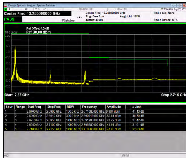
Band41_20MHz_QPSK_41490_1RB#0
