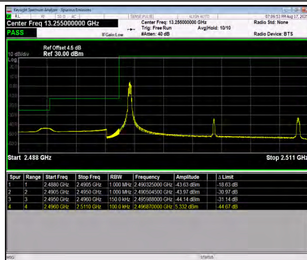
Band41_15MHz_QPSK_39725_1RB#0
