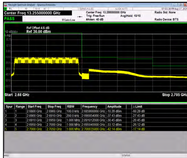
Band41_10MHz_QPSK_41540_50RB#0
