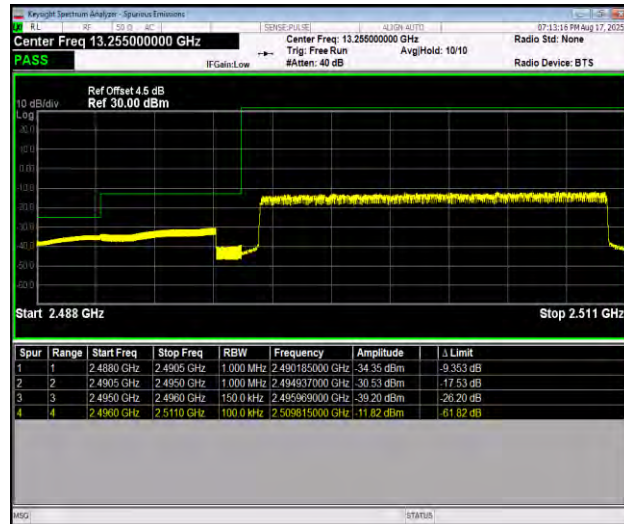
Band41_15MHz_QPSK_39725_75RB#0
