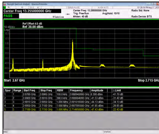
Band41_20MHz_QPSK_41490_1RB#99
