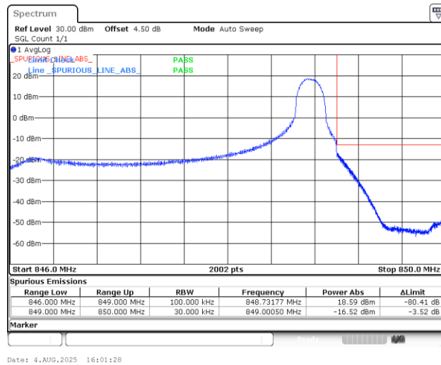
Band5_3MHz_16QAM_20635_1RB#14
