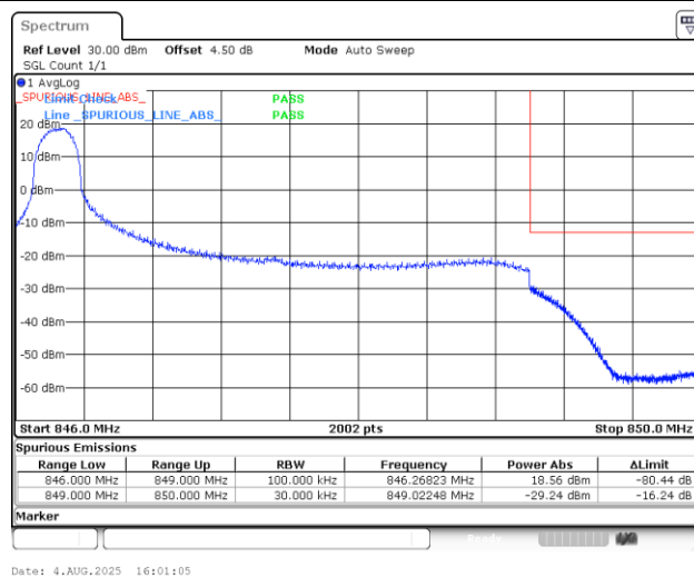
Band5_3MHz_16QAM_20635_1RB#0
