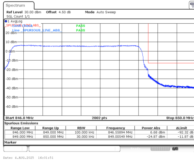
Band5_3MHz_16QAM_20635_15RB#0
