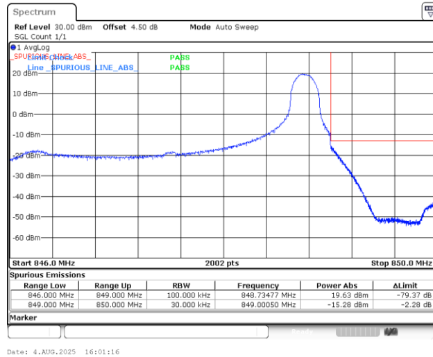
Band5_3MHz_QPSK_20635_1RB#14
