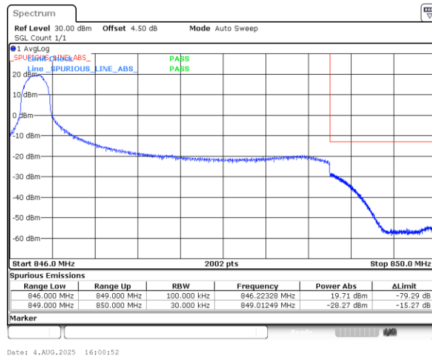
Band5_3MHz_QPSK_20635_1RB#0
