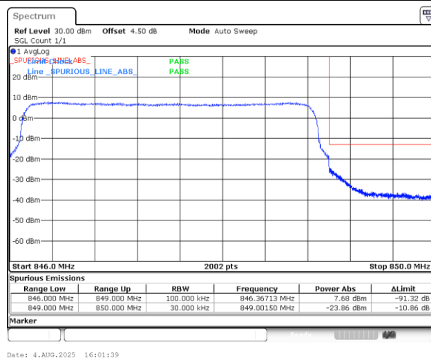
Band5_3MHz_QPSK_20635_15RB#0
