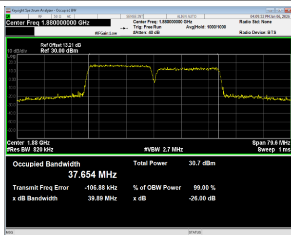
2C 64QAM PCC BW=20MHz Ch=801 RB=100@0,SCC BW=20MHz Ch=999 RB=100@0
