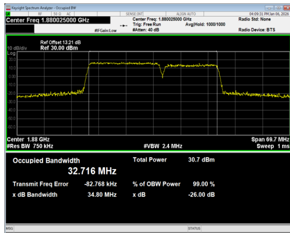
2C 64QAM PCC BW=20MHz Ch=826 RB=100@0,SCC BW=15MHz Ch=997 RB=75@0
