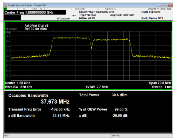
2C 16QAM PCC BW=20MHz Ch=801 RB=100@0,SCC BW=20MHz Ch=999 RB=100@0
