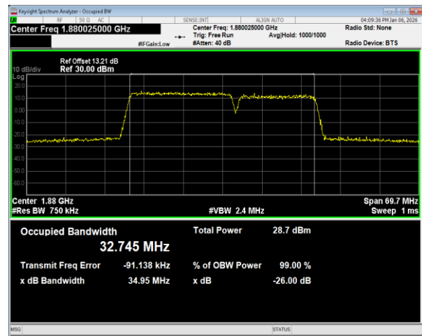
2C 256QAM PCC BW=20MHz Ch=826 RB=100@0,SCC BW=15MHz Ch=997 RB=75@0
