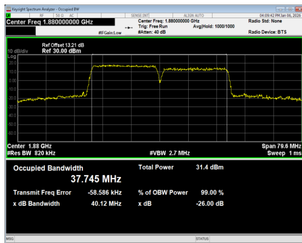
2C QPSK PCC BW=20MHz Ch=801 RB=100@0,SCC BW=20MHz Ch=999 RB=100@0
