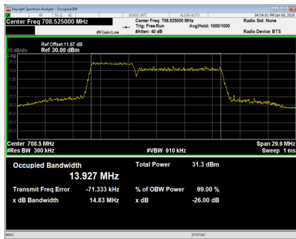
12B QPSK PCC BW=5MHz Ch=5058 RB=25@0,SCC BW=10MHz Ch=5130 RB=50@0
