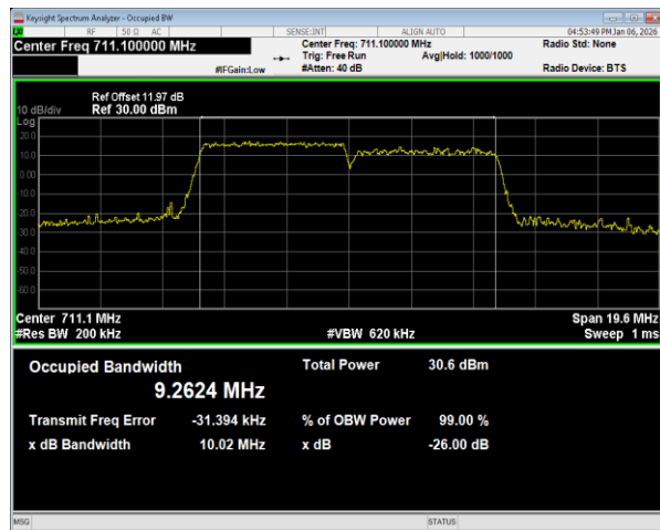
12B 64QAM PCC BW=5MHz Ch=5107 RB=25@0,SCC BW=5MHz Ch=5155 RB=25@0
