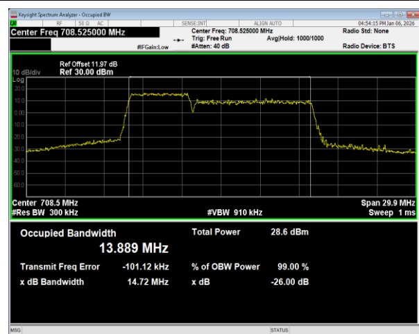
12B 256QAM PCC BW=5MHz Ch=5058 RB=25@0,SCC BW=10MHz Ch=5130 RB=50@0
