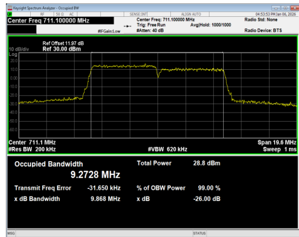
12B 256QAM PCC BW=5MHz Ch=5107 RB=25@0,SCC BW=5MHz Ch=5155 RB=25@0
