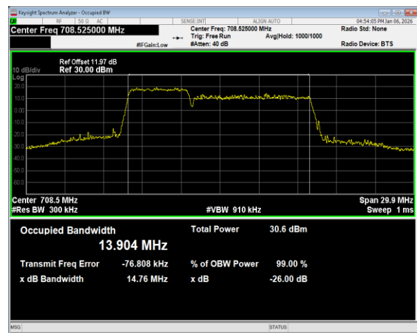
12B 16QAM PCC BW=5MHz Ch=5058 RB=25@0,SCC BW=10MHz Ch=5130 RB=50@0
