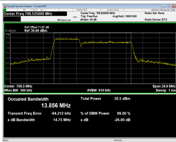
12B 64QAM PCC BW=5MHz Ch=5058 RB=25@0,SCC BW=10MHz Ch=5130 RB=50@0
