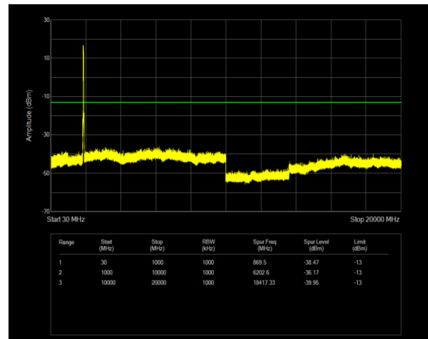
2C QPSK PCC BW=20MHz Ch=801 RB=100@0,SCC BW=20MHz Ch=999 RB=100@0
