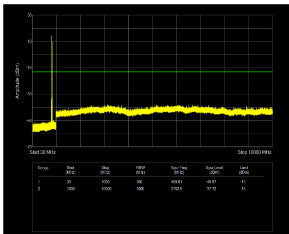
5B QPSK PCC BW=10MHz Ch=2501 RB=1@0,SCC BW=10MHz Ch=2600 RB=1@49
