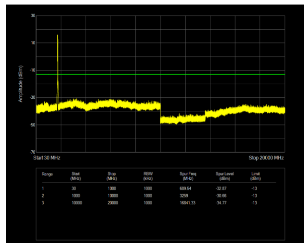
66C QPSK PCC BW=20MHz Ch=66787 RB=100@0,SCC BW=20MHz Ch=66985 RB=100@0
