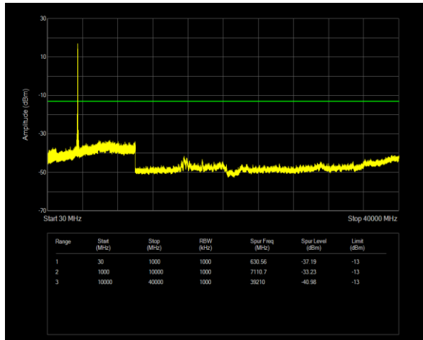
42C(3450-3550) QPSK PCC BW=20MHz Ch=42190 RB=1@0,SCC BW=20MHz Ch=42388 RB=1@99
