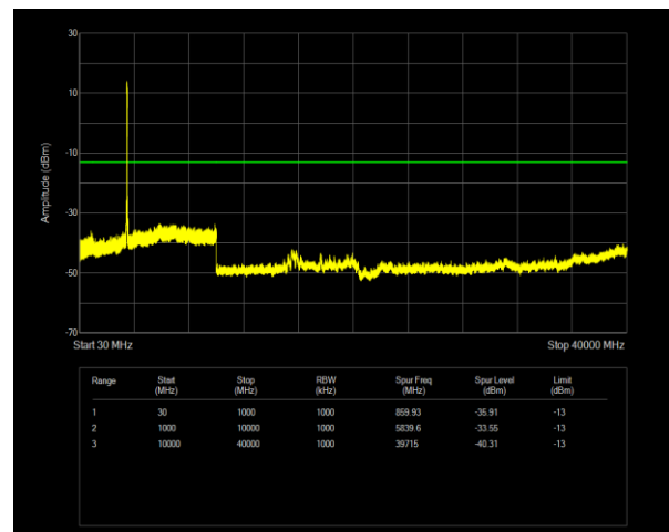
42C(3450-3550) QPSK PCC BW=20MHz Ch=42491 RB=100@0,SCC BW=20MHz Ch=42689 RB=100@0
