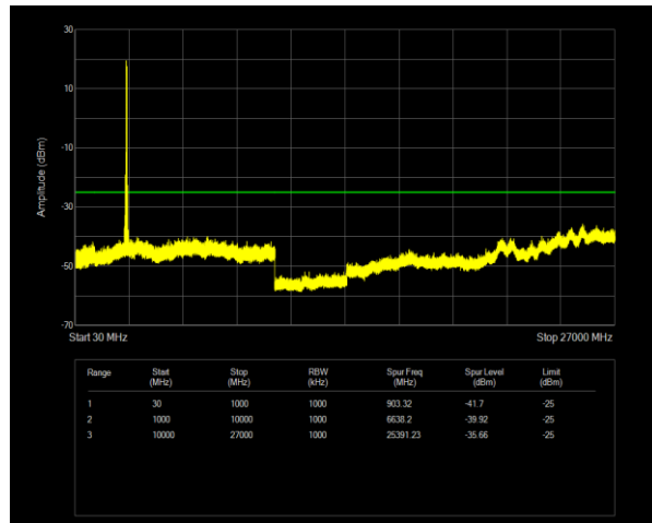
38C QPSK PCC BW=20MHz Ch=37850 RB=1@0,SCC BW=20MHz Ch=38048 RB=1@99
