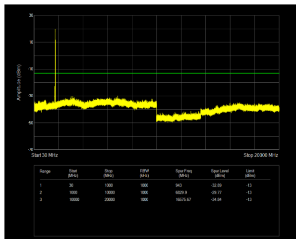
66C QPSK PCC BW=20MHz Ch=66787 RB=1@0,SCC BW=20MHz Ch=66985 RB=1@99
