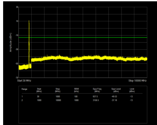
5B QPSK PCC BW=10MHz Ch=2450 RB=50@0,SCC BW=10MHz Ch=2549 RB=50@0
