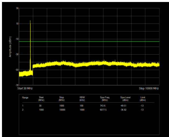
5B QPSK PCC BW=10MHz Ch=2476 RB=1@0,SCC BW=10MHz Ch=2575 RB=1@49
