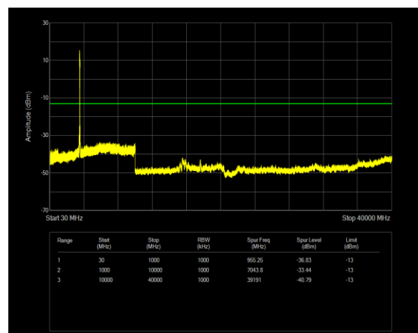
42C(3450-3550) QPSK PCC BW=20MHz Ch=42792 RB=100@0,SCC BW=20MHz Ch=42990 RB=100@0
