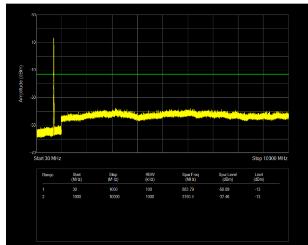
12B QPSK PCC BW=5MHz Ch=5038 RB=25@0,SCC BW=10MHz Ch=5110 RB=50@0
