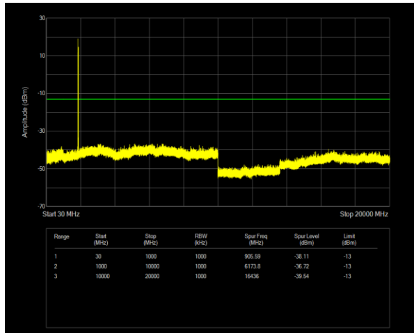
2C QPSK PCC BW=20MHz Ch=700 RB=1@0,SCC BW=20MHz Ch=898 RB=1@99
