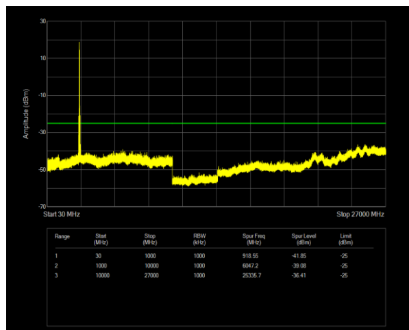
38C QPSK PCC BW=20MHz Ch=37901 RB=1@0,SCC BW=20MHz Ch=38099 RB=1@99
