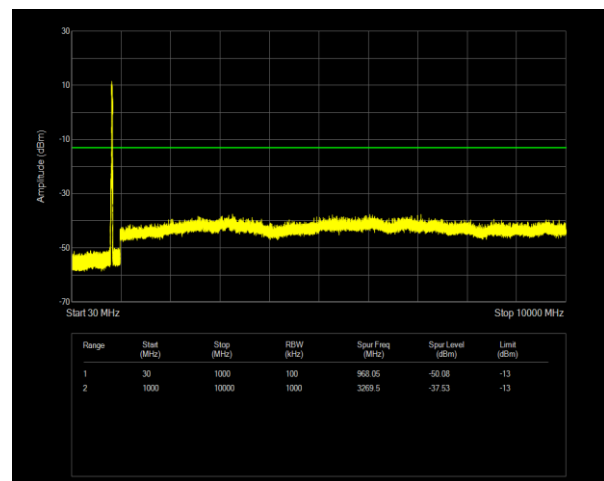
5B QPSK PCC BW=10MHz Ch=2501 RB=50@0,SCC BW=10MHz Ch=2600 RB=50@0
