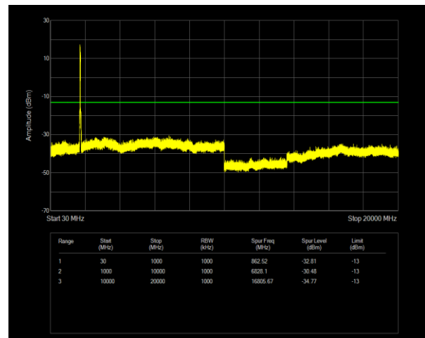
66C QPSK PCC BW=20MHz Ch=66536 RB=100@0,SCC BW=20MHz Ch=66734 RB=100@0
