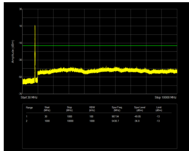
5B QPSK PCC BW=10MHz Ch=2476 RB=50@0,SCC BW=10MHz Ch=2575 RB=50@0
