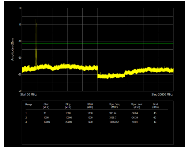
2C QPSK PCC BW=20MHz Ch=700 RB=100@0,SCC BW=20MHz Ch=898 RB=100@0
