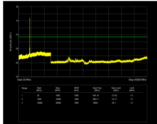
42C(3450-3550) QPSK PCC BW=20MHz Ch=42190 RB=100@0,SCC BW=20MHz Ch=42388 RB=100@0
