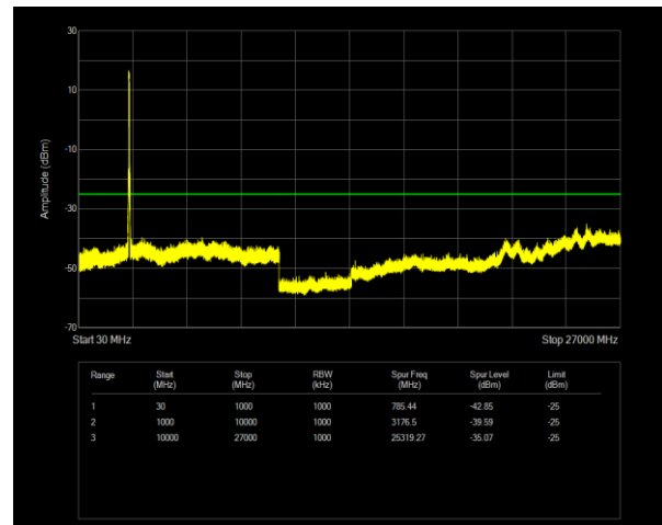
7C QPSK PCC BW=20MHz Ch=3001 RB=100@0,SCC BW=20MHz Ch=3199 RB=100@0
