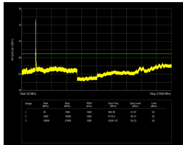
41C QPSK PCC BW=20MHz Ch=39750 RB=100@0,SCC BW=20MHz Ch=39948 RB=100@0
