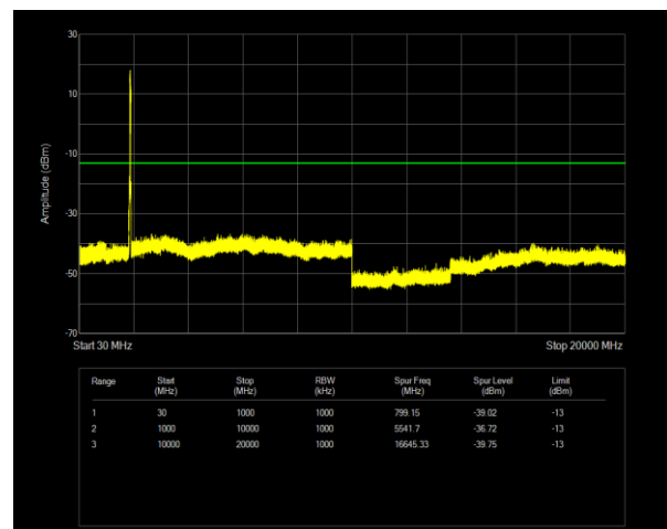
2C QPSK PCC BW=20MHz Ch=902 RB=100@0,SCC BW=20MHz Ch=1100 RB=100@0
