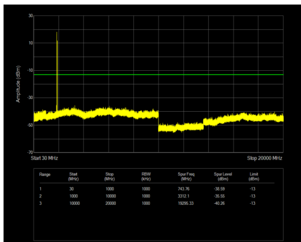
2C QPSK PCC BW=20MHz Ch=902 RB=1@0,SCC BW=20MHz Ch=1100 RB=1@99
