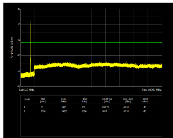
12B QPSK PCC BW=5MHz Ch=5058 RB=25@0,SCC BW=10MHz Ch=5130 RB=50@0
