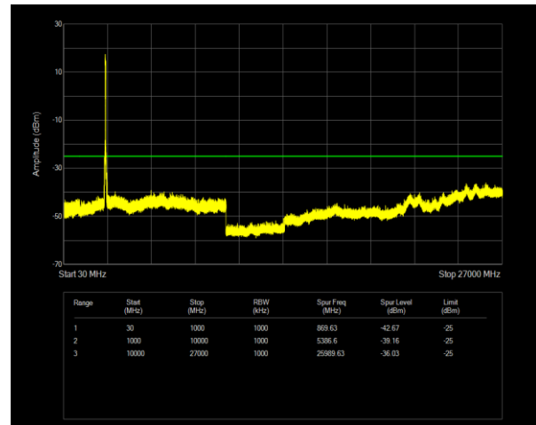
38C QPSK PCC BW=20MHz Ch=37850 RB=100@0,SCC BW=20MHz Ch=38048 RB=100@0
