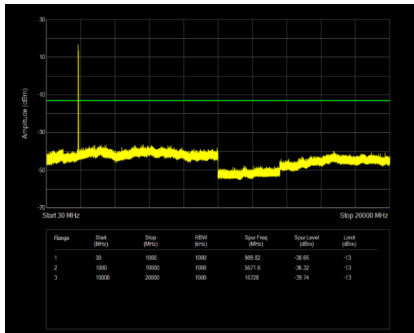
2C QPSK PCC BW=20MHz Ch=801 RB=1@0,SCC BW=20MHz Ch=999 RB=1@99
