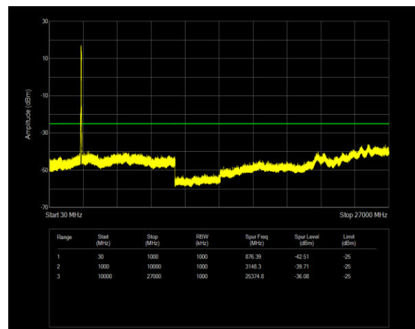
7C QPSK PCC BW=20MHz Ch=3152 RB=100@0,SCC BW=20MHz Ch=3350 RB=100@0
