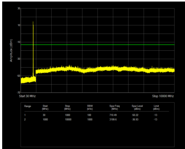
5B QPSK PCC BW=10MHz Ch=2450 RB=1@0,SCC BW=10MHz Ch=2549 RB=1@49
