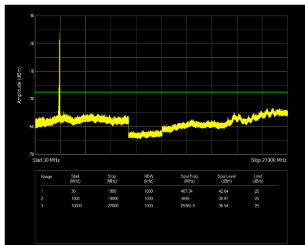
38C QPSK PCC BW=20MHz Ch=37952 RB=1@0,SCC BW=20MHz Ch=38150 RB=1@99
