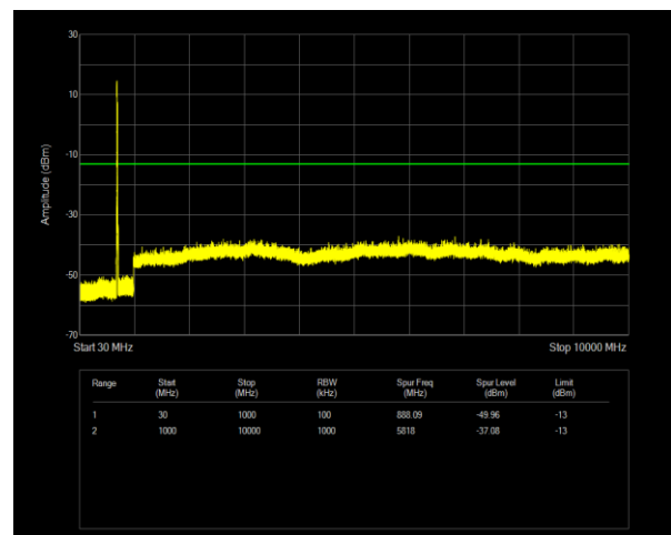
12B QPSK PCC BW=5MHz Ch=5048 RB=25@0,SCC BW=10MHz Ch=5120 RB=50@0
