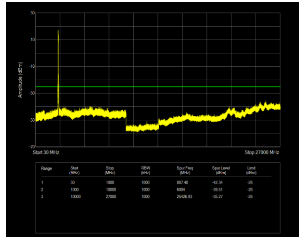
7C QPSK PCC BW=20MHz Ch=2850 RB=100@0,SCC BW=20MHz Ch=3048 RB=100@0
