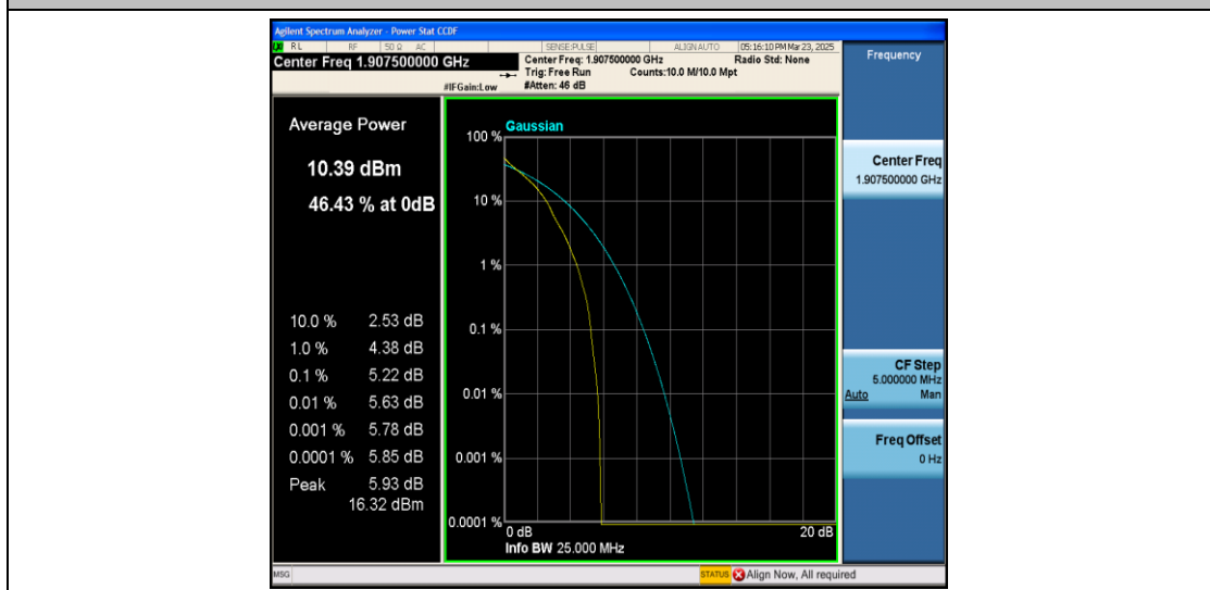
Band2-5MHz-QPSK-19175-1RB#0-PASS
