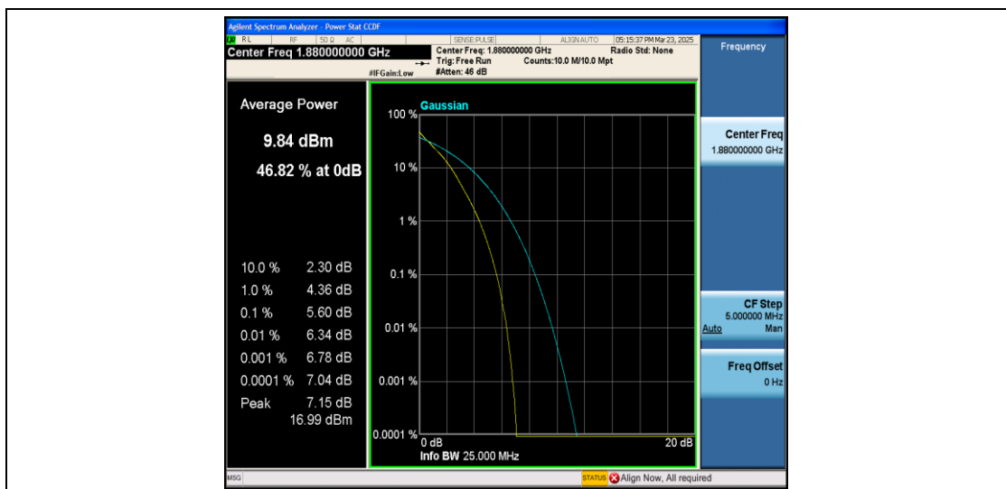
Band2-5MHz-QPSK-18900-25RB#0-PASS
