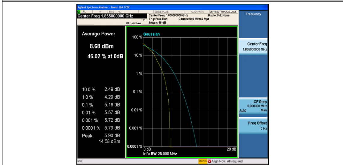
Band2-10MHz-QPSK-18650-1RB#0-PASS
