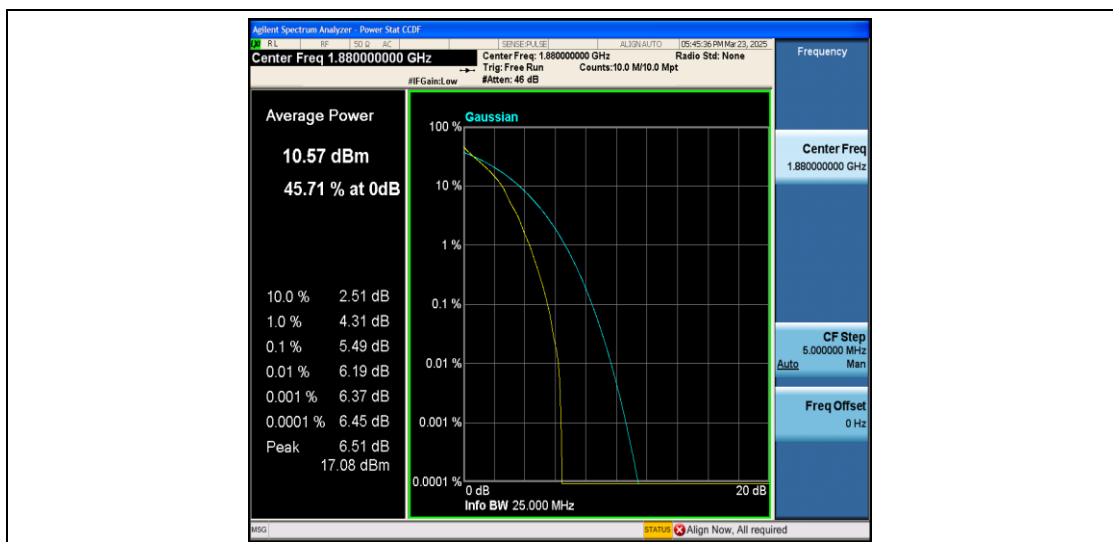
Band2-10MHz-QPSK-18900-1RB#0-PASS
