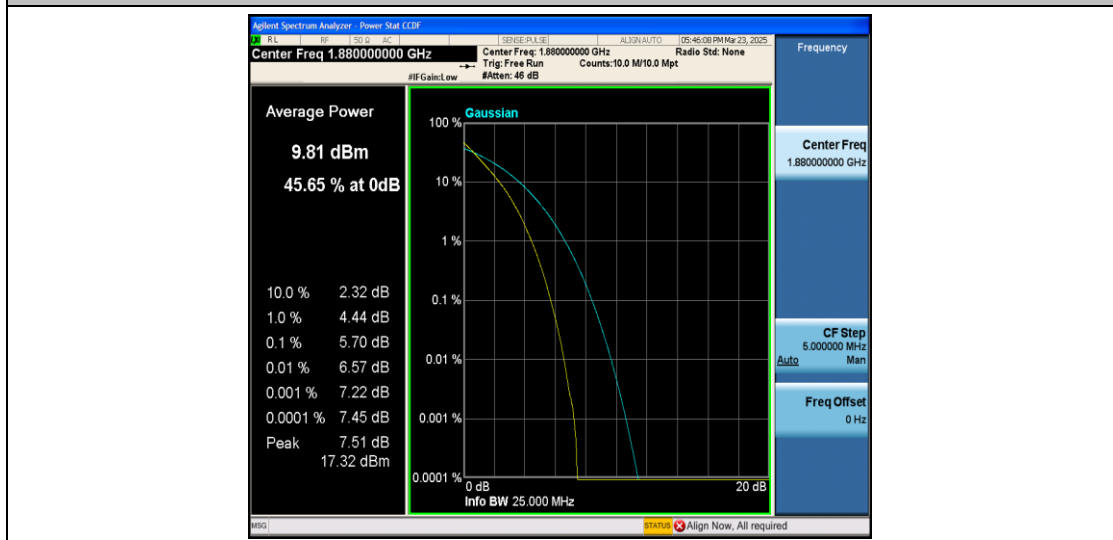
Band2-10MHz-QPSK-18900-50RB#0-PASS
