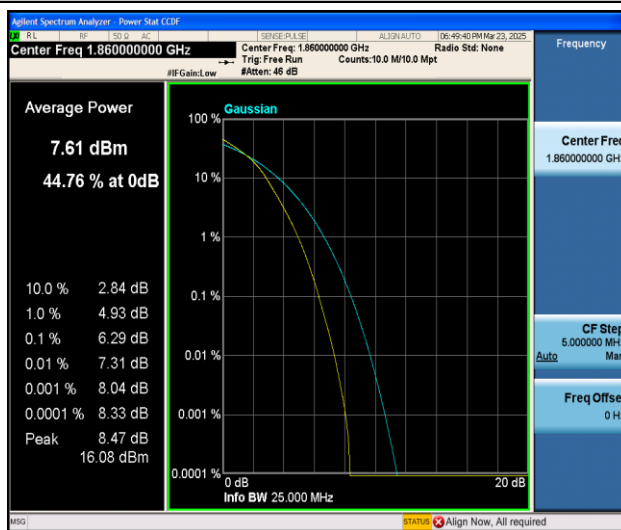
Band2-20MHz-16QAM-18700-100RB#0-PASS
