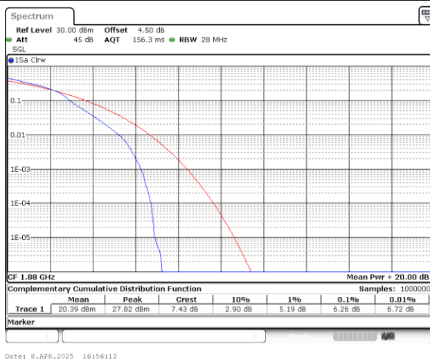
Band2-20MHz-16QAM-18900-1RB#0-PASS
