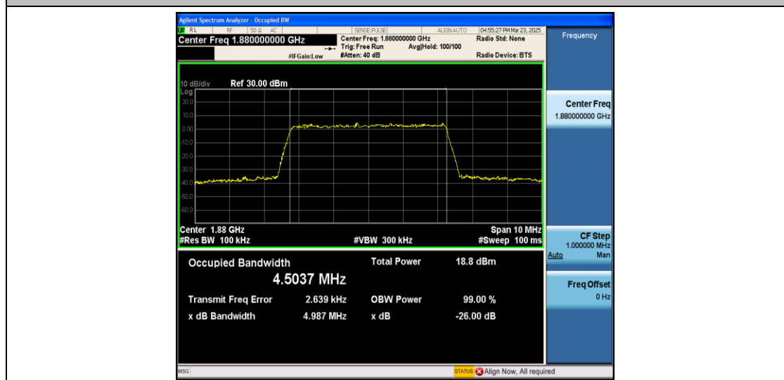
Band2-5MHz-QPSK-18900-25RB#0-PASS
