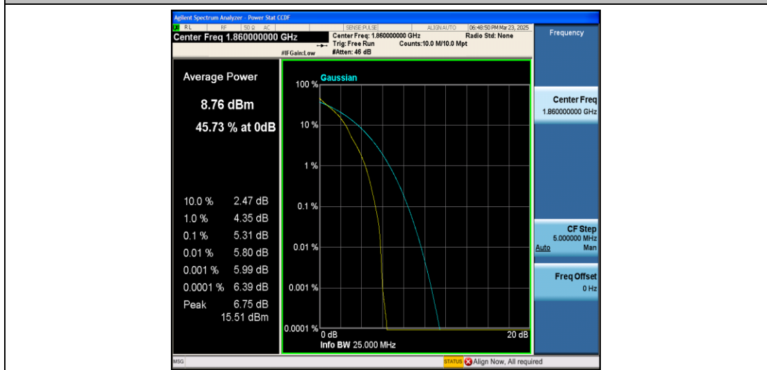
Band2-20MHz-QPSK-18700-1RB#0-PASS
