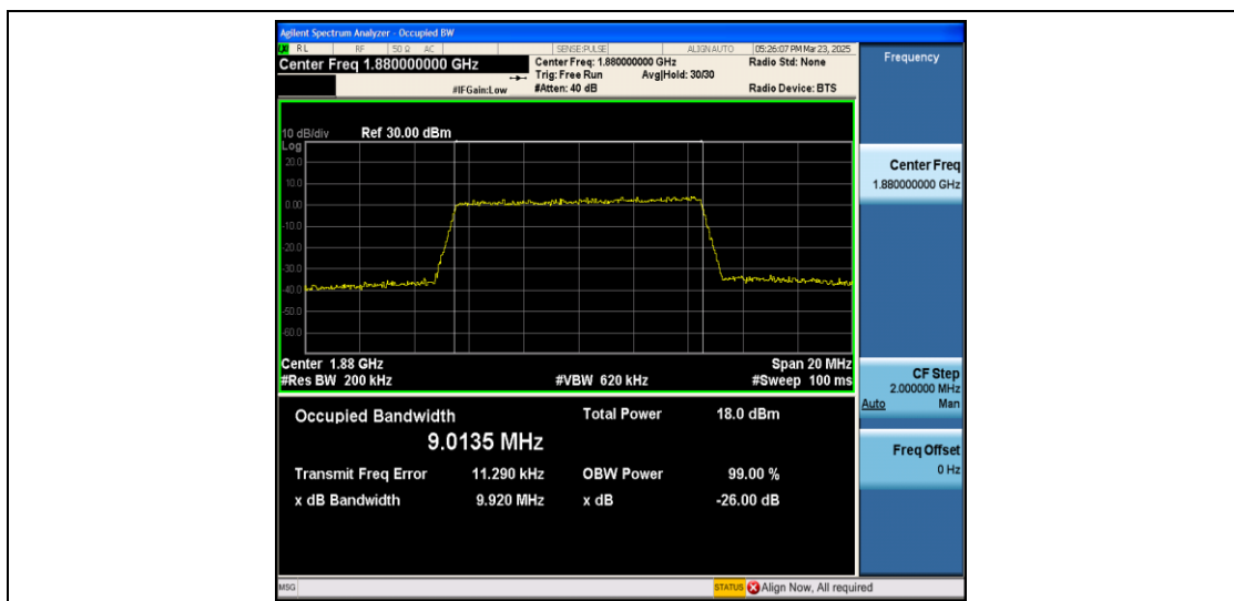
Band2-10MHz-16QAM-18900-50RB#0-PASS
