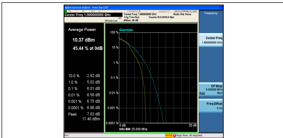
Band2-20MHz-16QAM-19100-1RB#0-PASS
