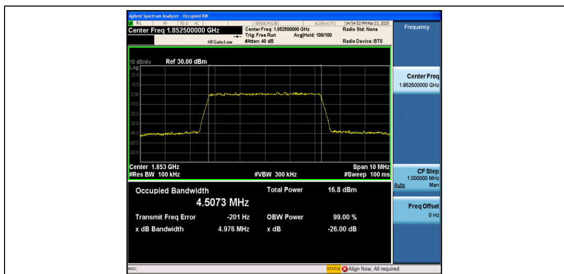
Band2-5MHz-QPSK-18625-25RB#0-PASS
