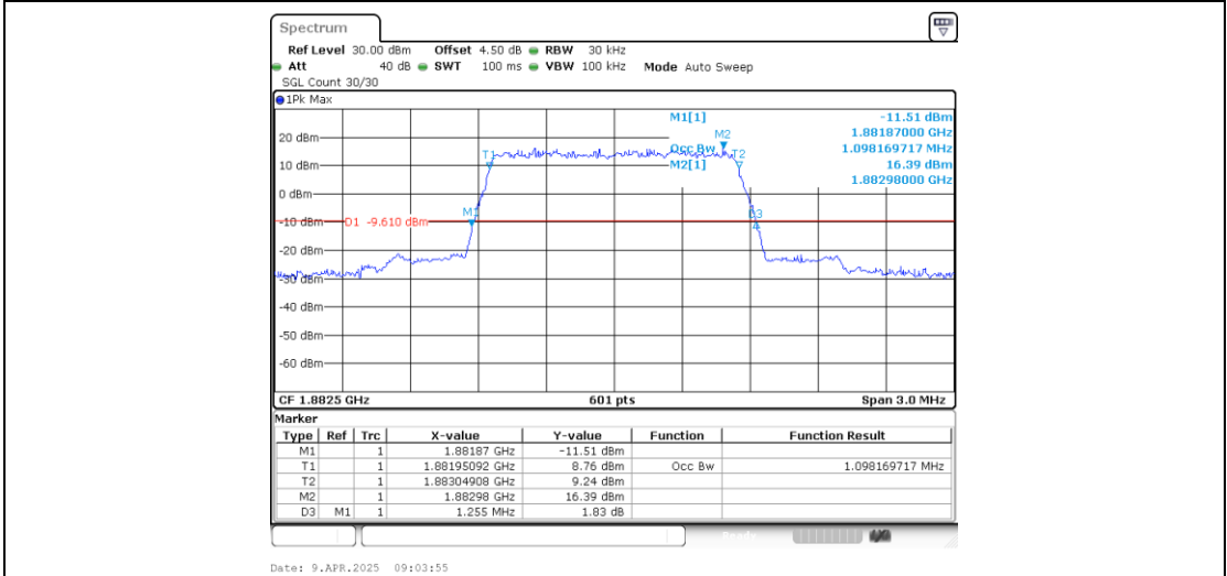
Band25-1.4MHz-QPSK-26365-6RB#0-PASS
