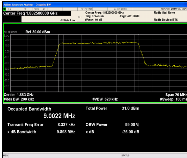
Band25-10MHz-QPSK-26365-50RB#0-PASS
