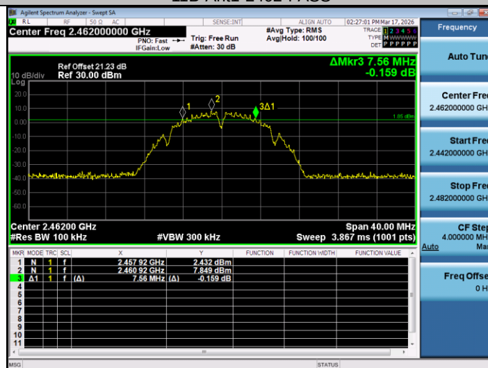
11B-Ant2-2462-PASS
