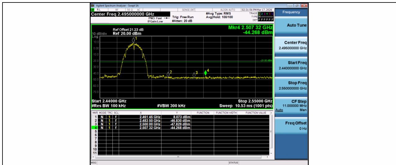
11B-Ant2-2462-PASS
