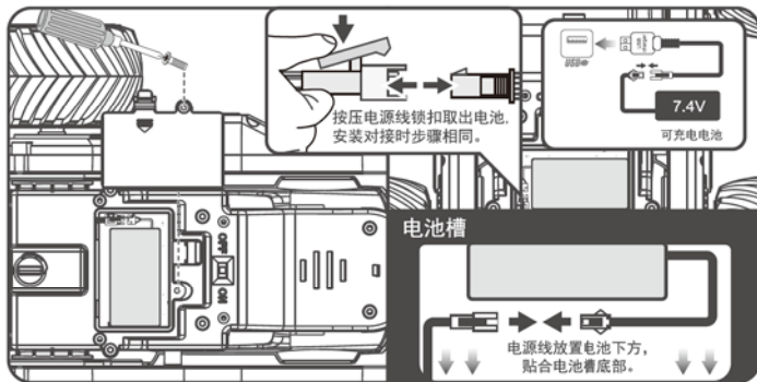
车体装入电池示意图
