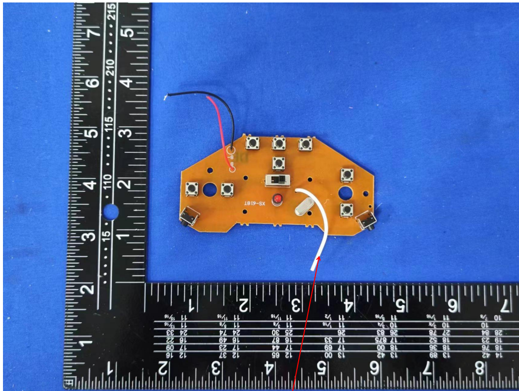
2.4G ANT
