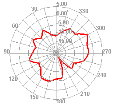
2400.000MHz E1
