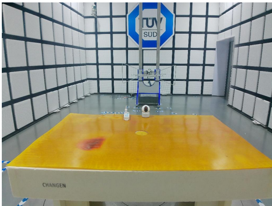
30MHz-1000MHz RSE Setup
