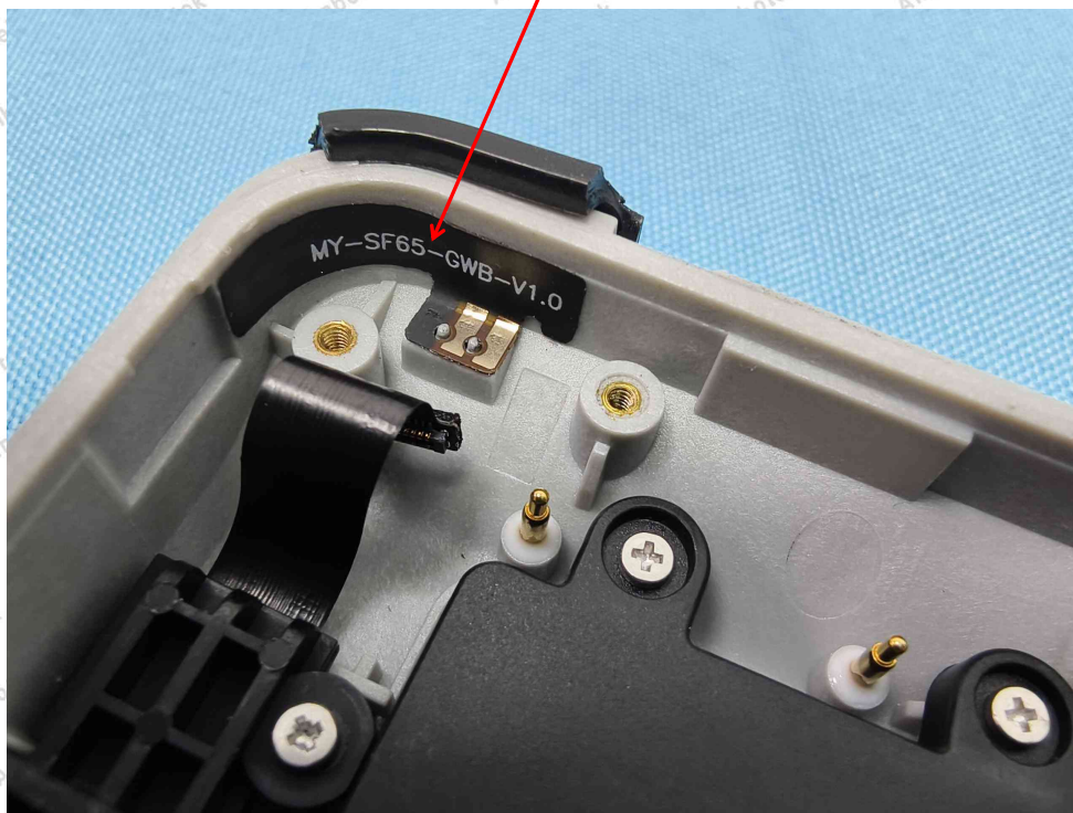
BT+WIFI+GPS ANT
