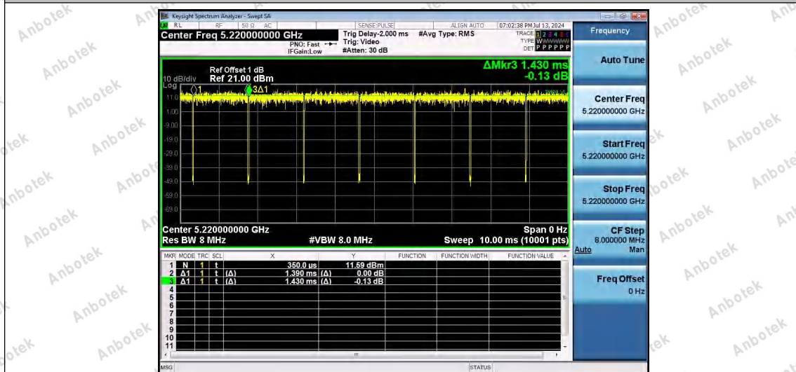
NTNV-11A-Ant1-5220
