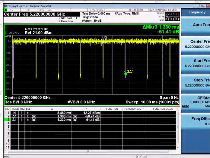
NTNV-11N20SISO-Ant1-5220
